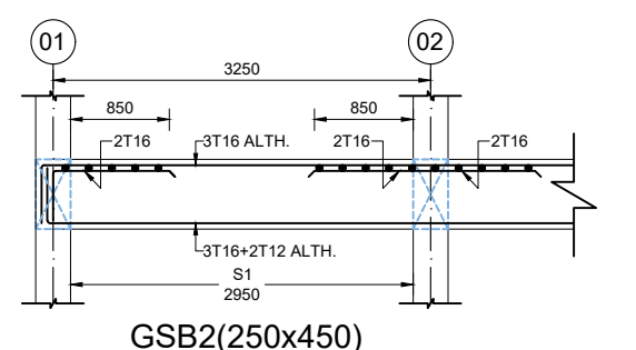
PB2(250x450)
