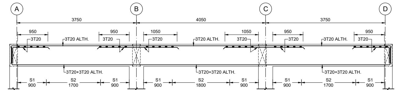
TB9(250x700)
