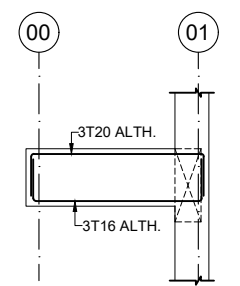
TB2(250x450)
