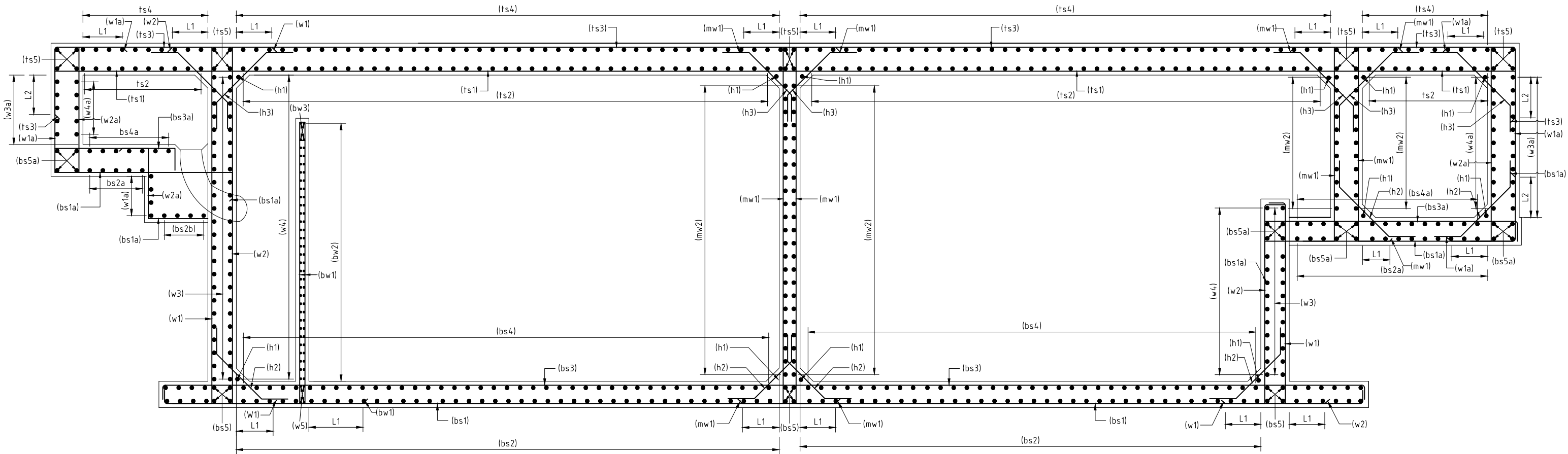
SECTION A-A SCALE : 1/30
